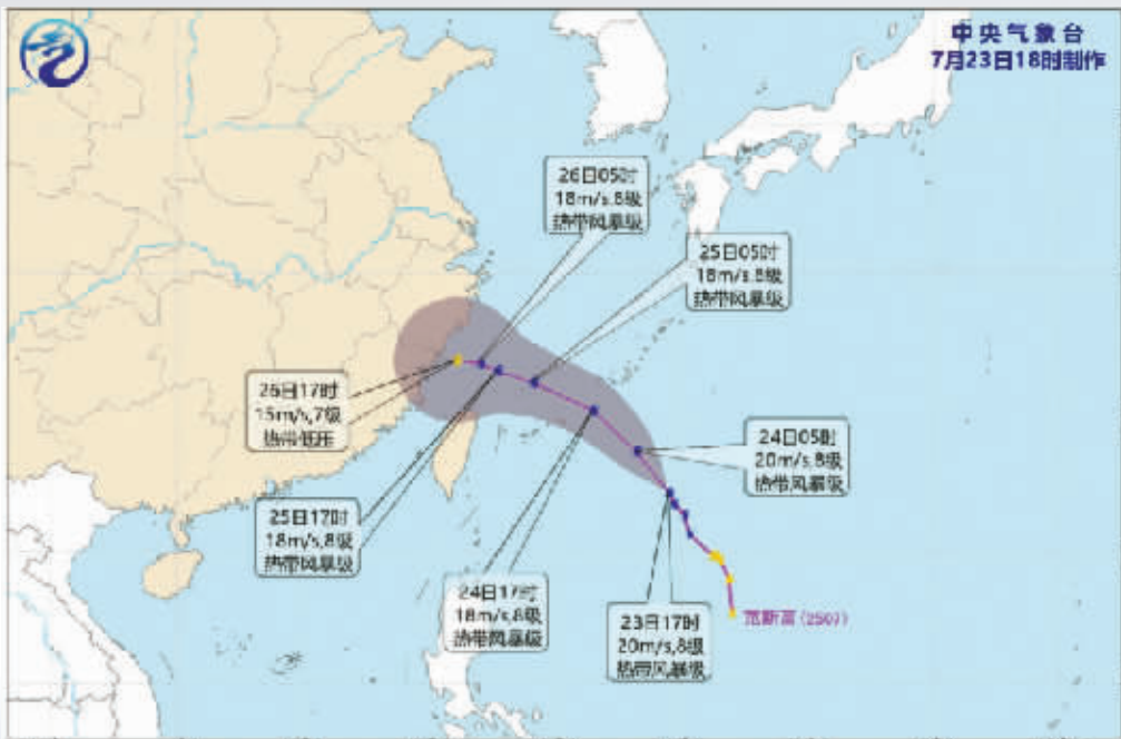
“范斯高”未来72小时路径概率预报图
