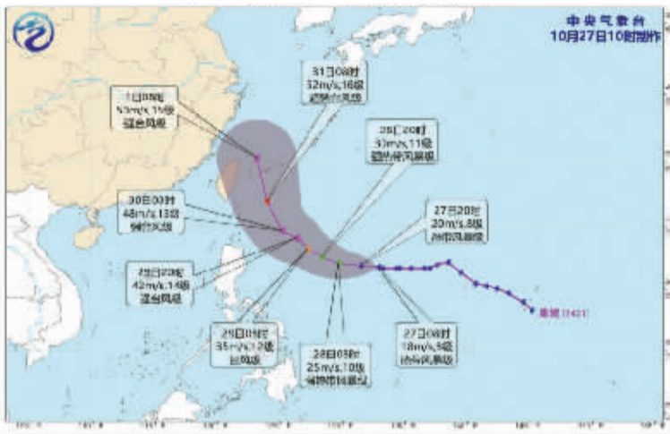
今年第21号台风“康妮”未来120小时路径概率预报图 2024年10月27日08时-11月1日08时(北京时间)
