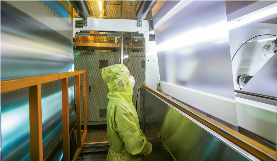
激智科技生产车间。
