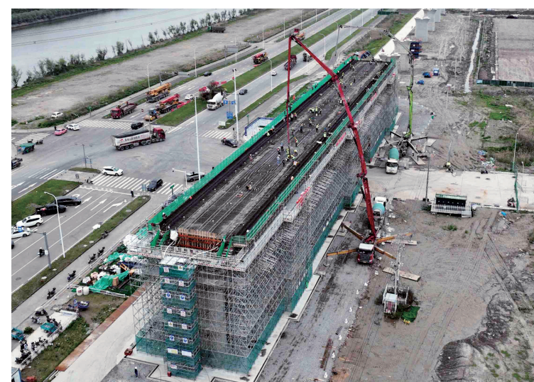
前晚8时18分，在前湾新区龙宝路东侧施工现场，经过20个小时连续奋战，通苏嘉甬高铁特大桥A段首联连续梁浇筑完成，标志着桥梁上部结构施工正式拉开序幕，项目建设全面开启加速度。（徐能 虞昌胜 摄）
